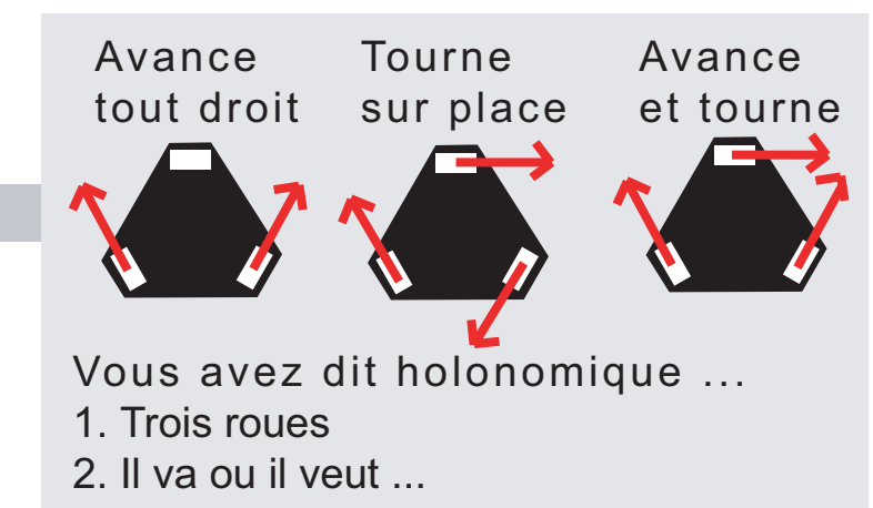
Roues omnidirectionnelles
